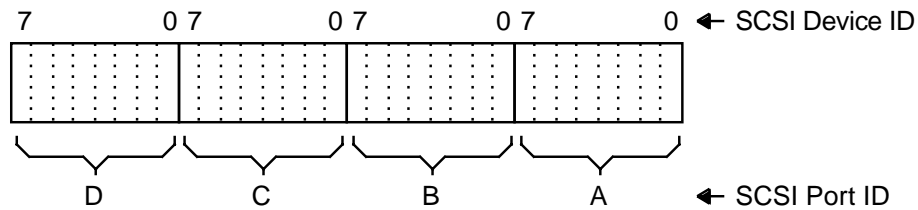
Figure 8-3 SCSI_NOAUTO System Parameter
